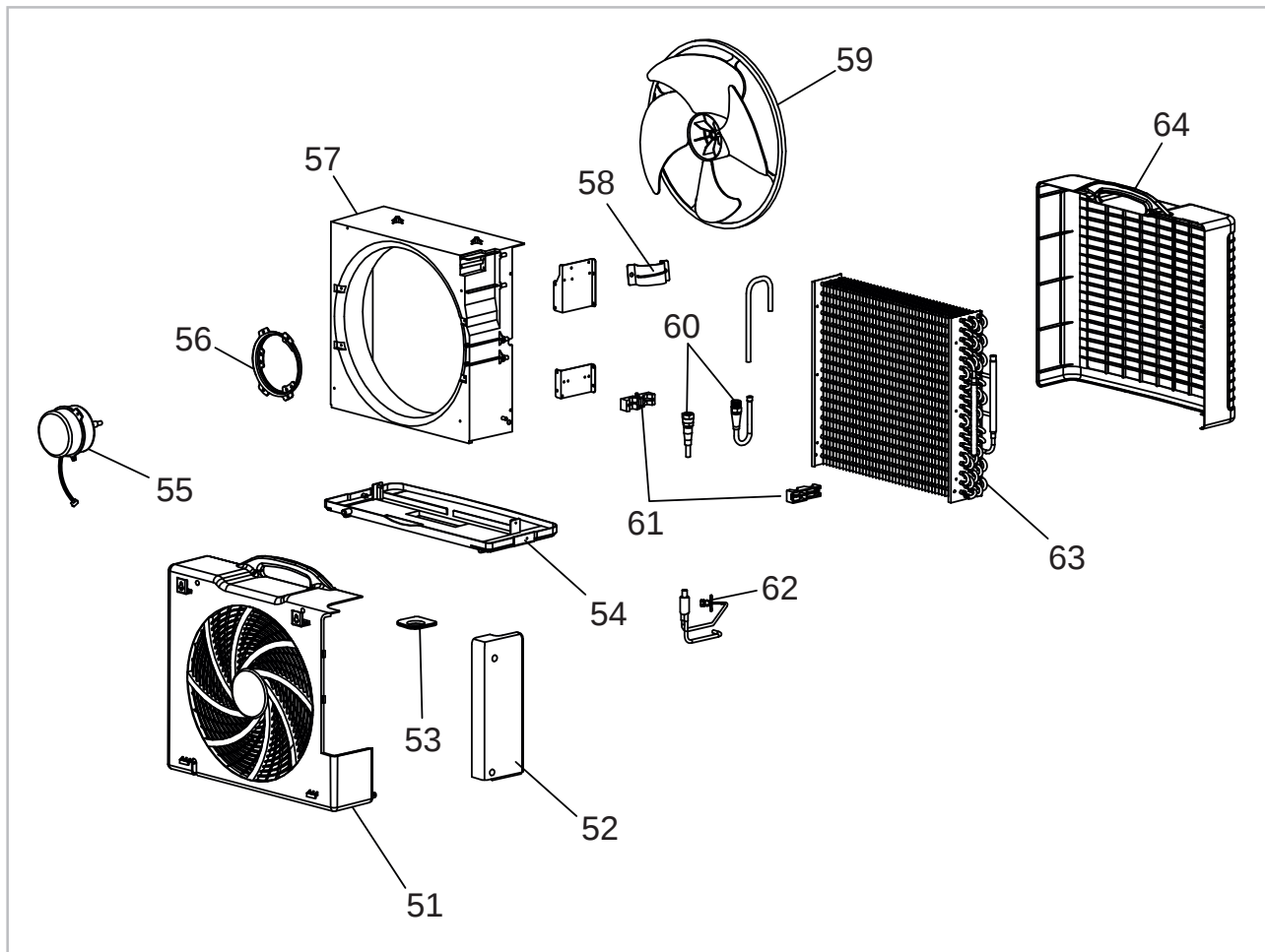
Abb. 22: Explosionszeichnung Außenteil
