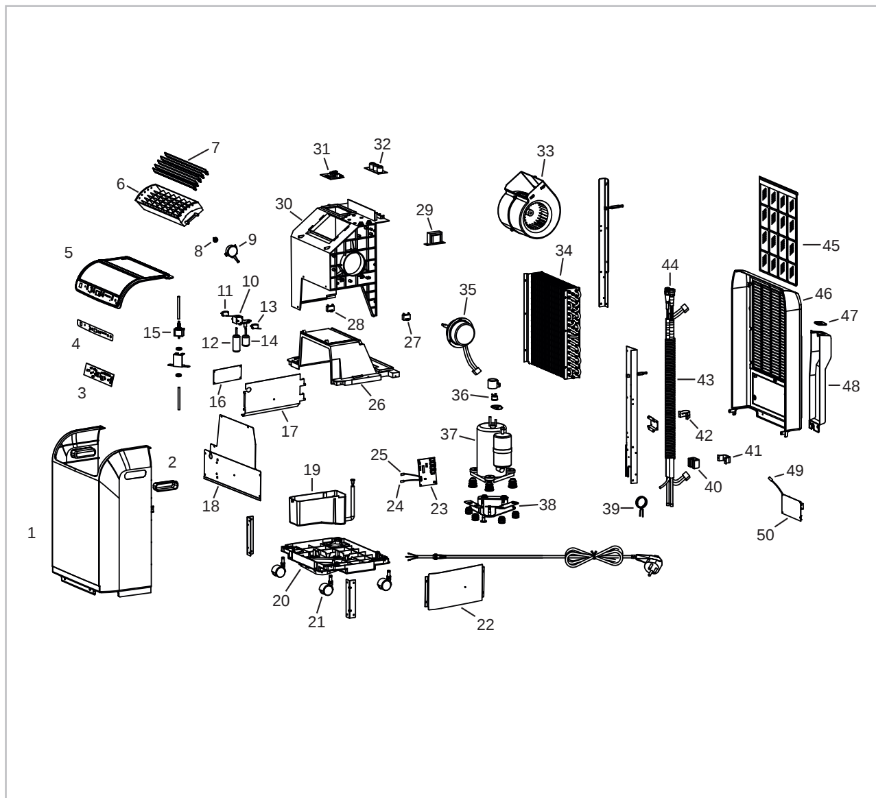
Abb. 21: Explosionszeichnung Innengerät
