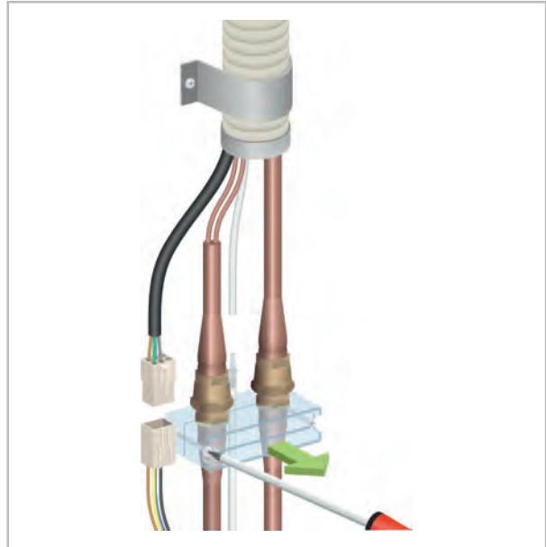
Abb. 16: Halterung entfernen
