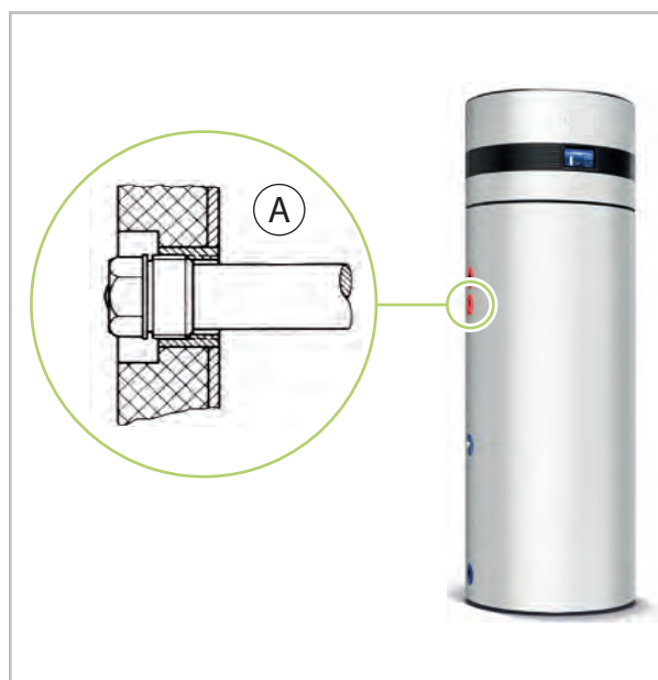
Abb. 4: Austausch der Magnesiumanode (450 mm)
