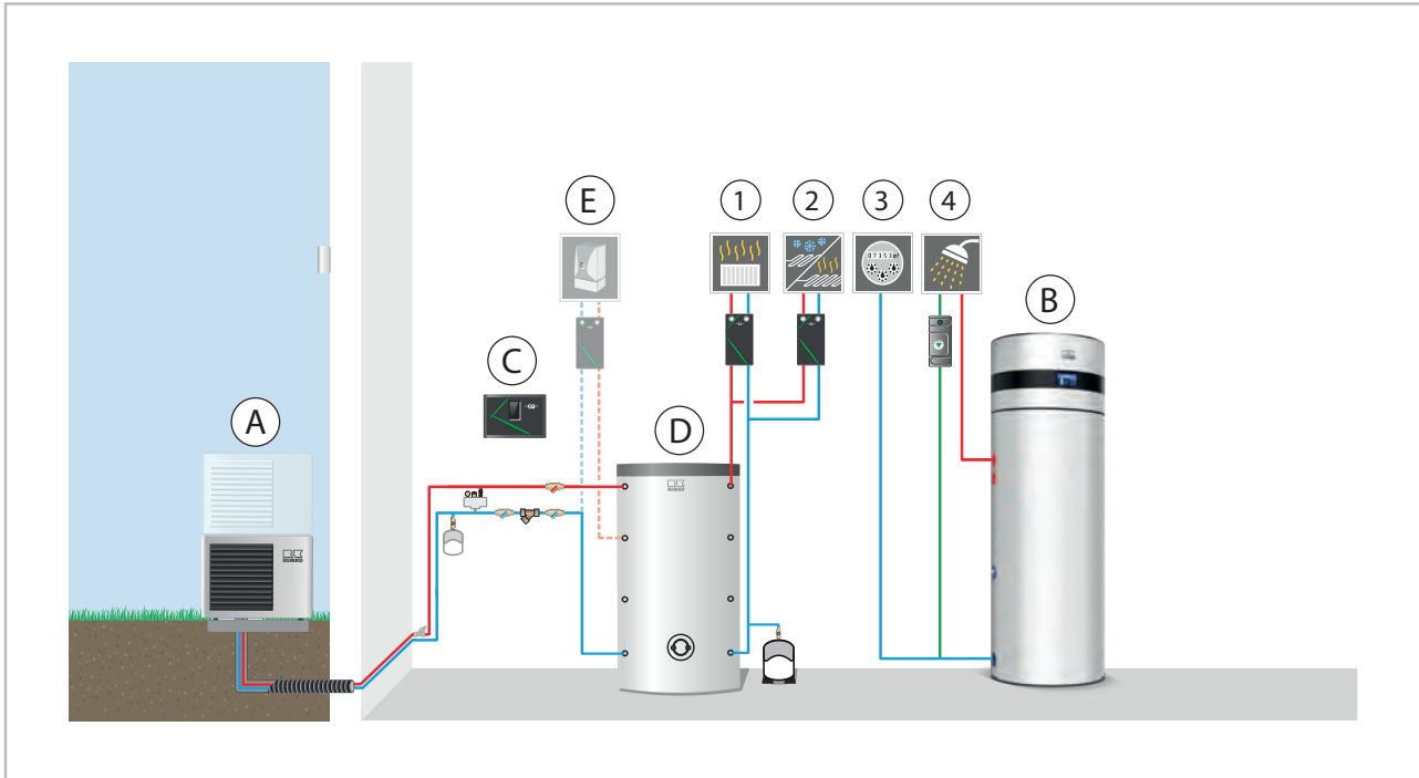
Abb. 12: Beispiel 1 - Hydraulikschema
