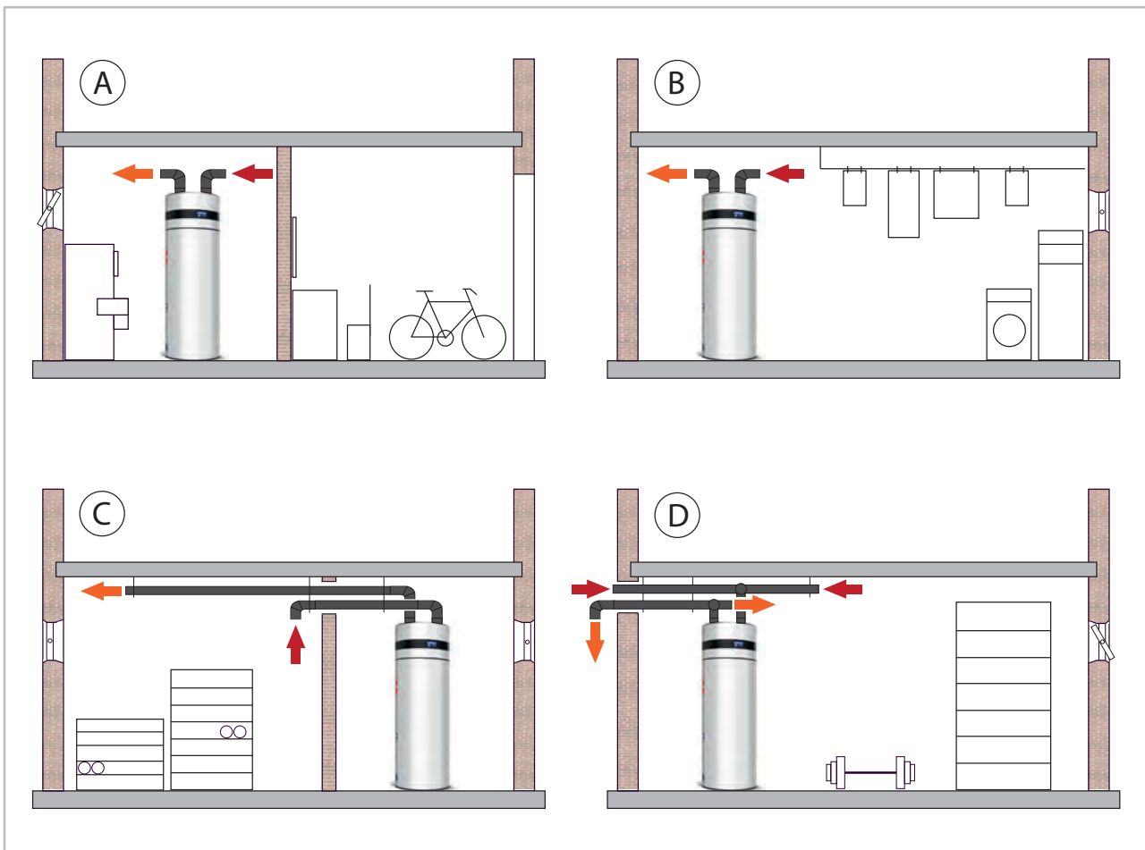
Abb. 10: Installationsmöglichkeiten
