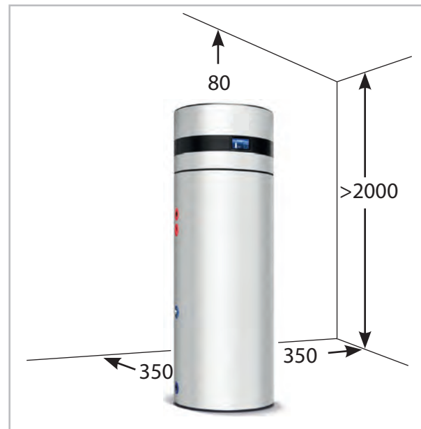
Abb. 8: Mindestabstände in mm
