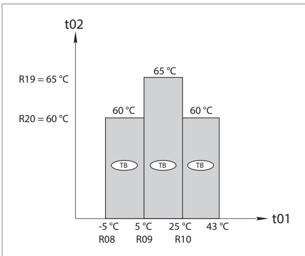
Abb. 19: Kontrolllogik Kompressor
