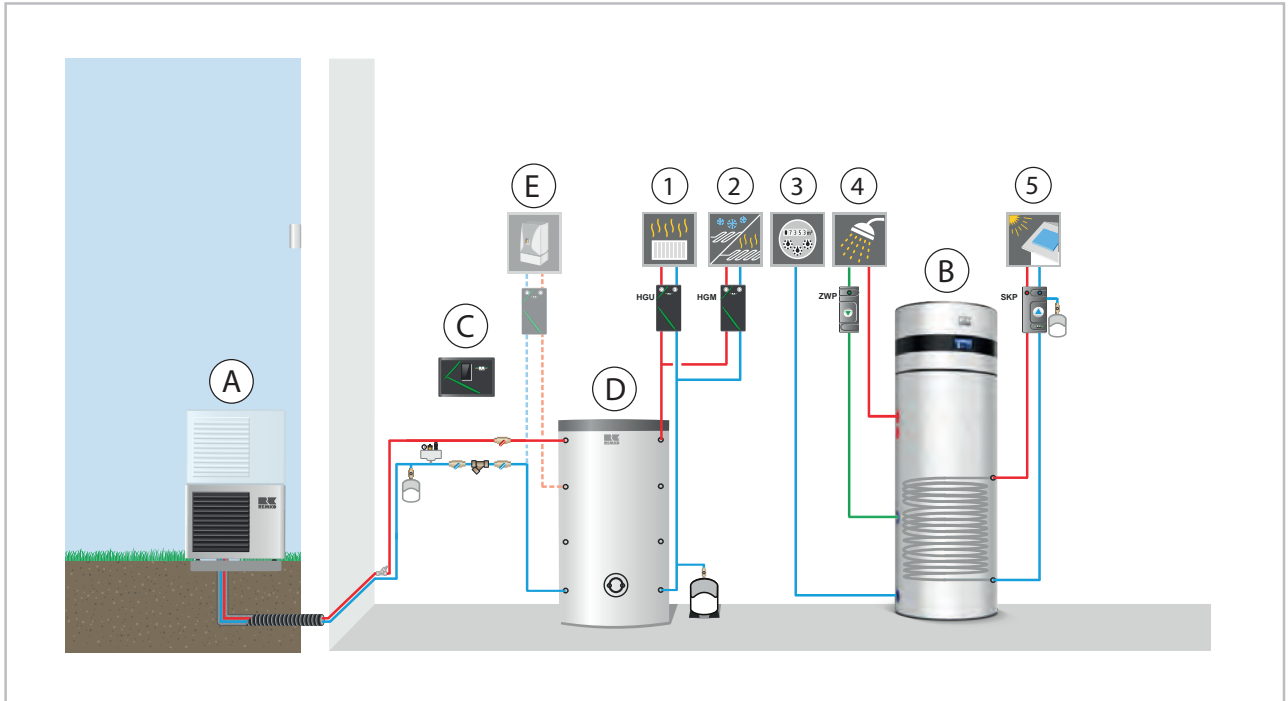
Abb. 13: Beispiel 2 - Hydraulikschema
