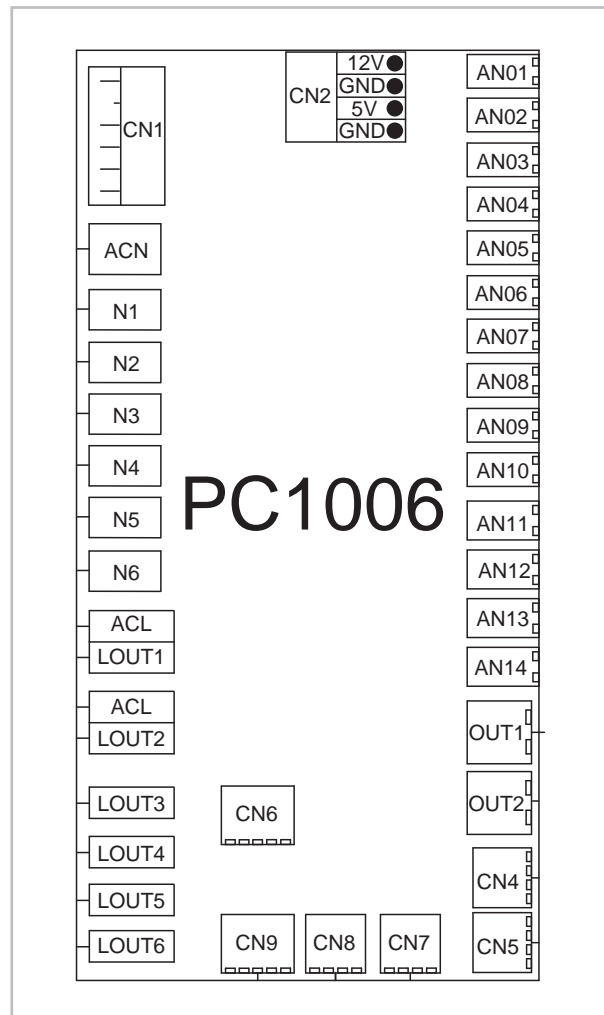
Abb. 14: Anschlüsse Leistungsplatine
